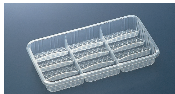
WG-12 サイズ:225×125×30(60L)mm 入数 1000 材質:PP 規格品 ㊦
